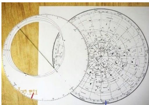
Пример звездной карты и накладного круга.
